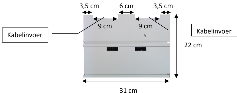
Linker zijaanzicht
