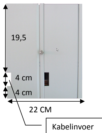
Linker zijaanzicht
